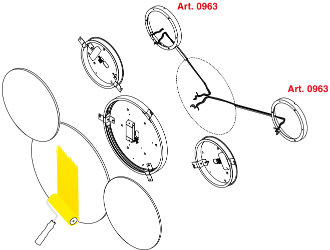
Esempio di installazione multipla con distanziali. Example of multiple installation with spacers.
