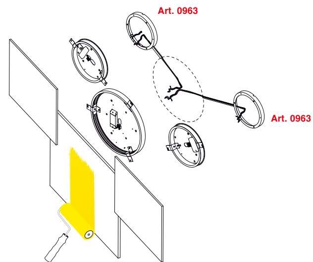
Esempio di installazione multipla con distanziali. Example of multiple installation with spacers.
