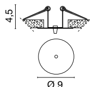
Piastra con molle per controsoffitti Ceiling plate with springs
